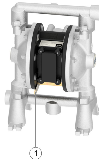
13. ábra: Földelés csatlakoztatása
