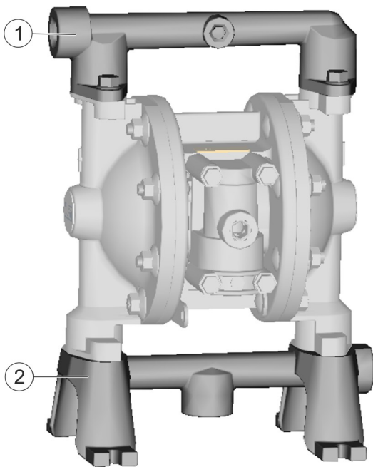
10. ábra: Be- és kimeneti gyűjtőcső, N24140009
