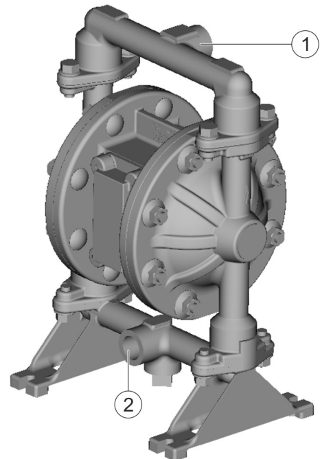
15. ábra: Anyagellátási csatlakozó, N24140007
