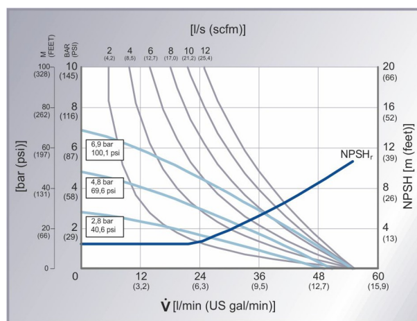
40. ábra: Kiáramlás sebesség diagram, N24140009
